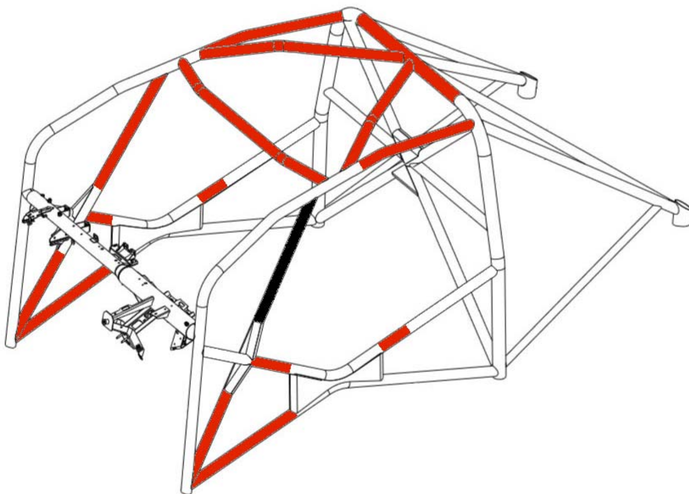
Figure 1 : Emplacements de la garniture d'arceau
